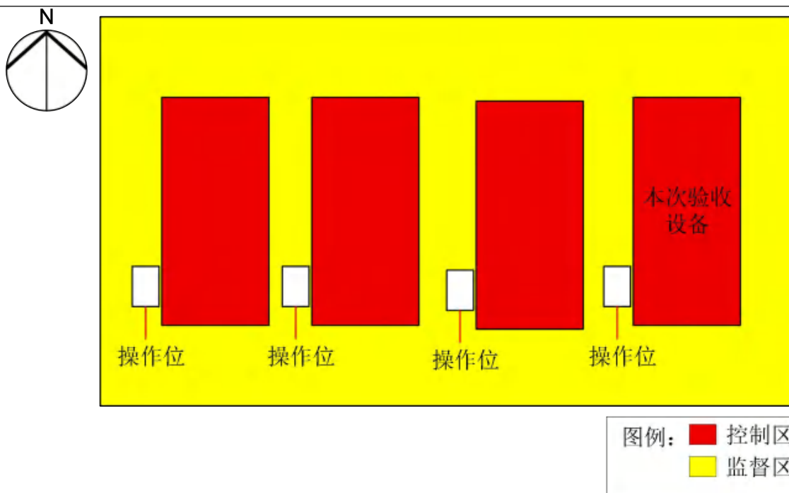
图2-5 CT检测区平面布置图
